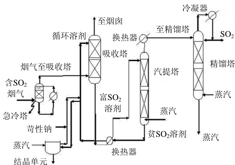
图 1 SolvR™二氧化硫回收系统简化工艺流程
